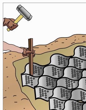
C Piquets bois
