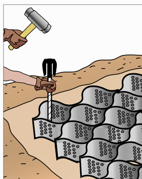
B Ancrages ATRA®
